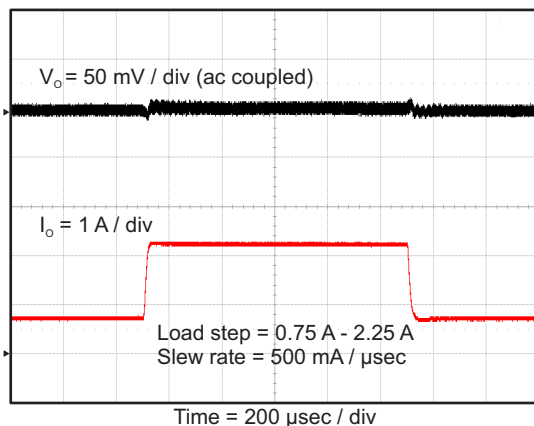
瞬态响应
